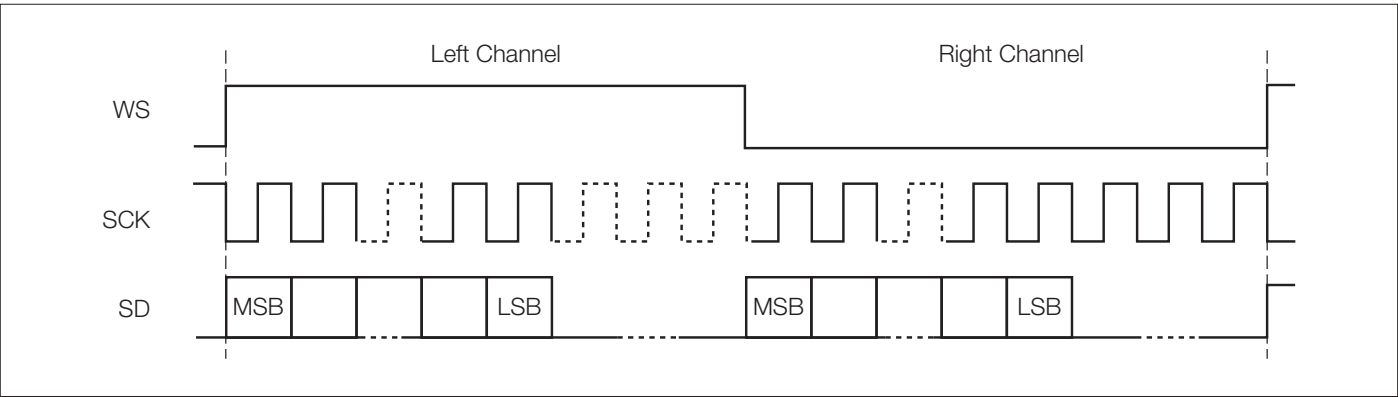
Figure 39 part II. LJ Format.
